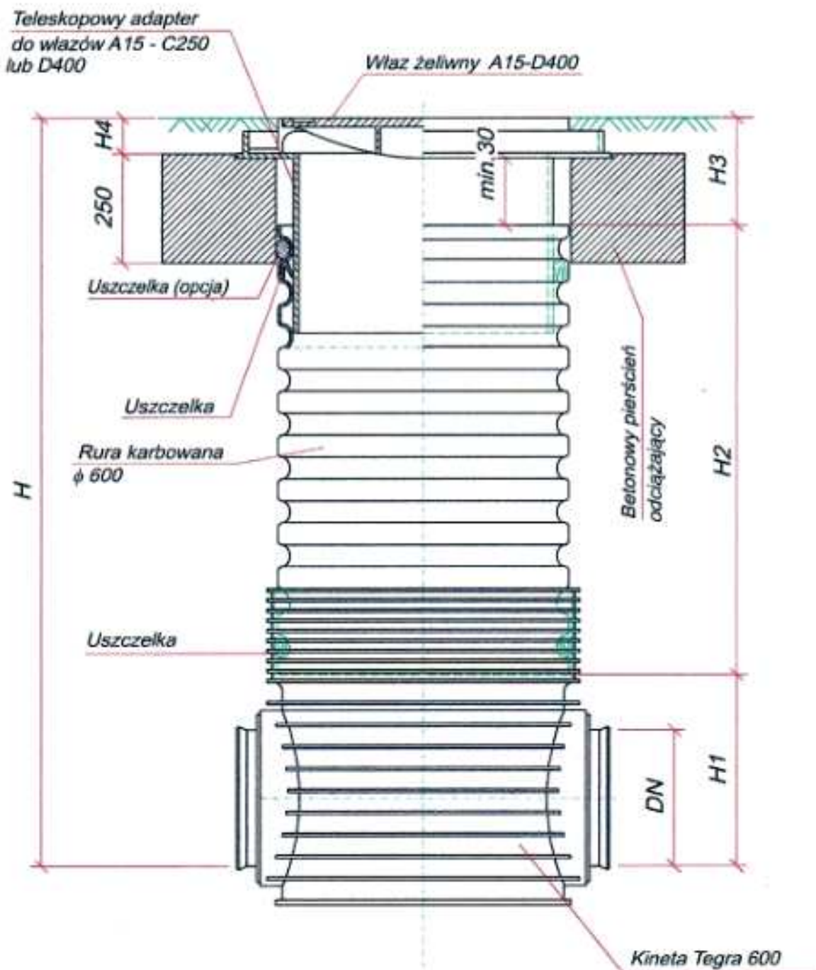
Rys 5. Schemat studzienki kanalizacyjnej DN600
